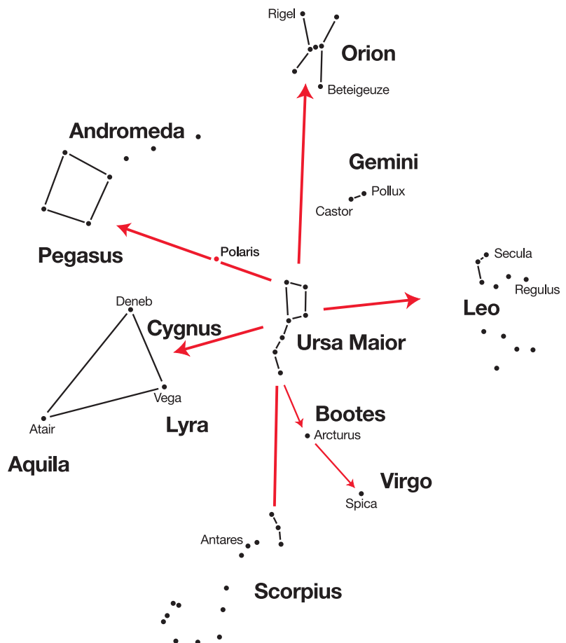
Abb. 48: Einfache Sternkarte
