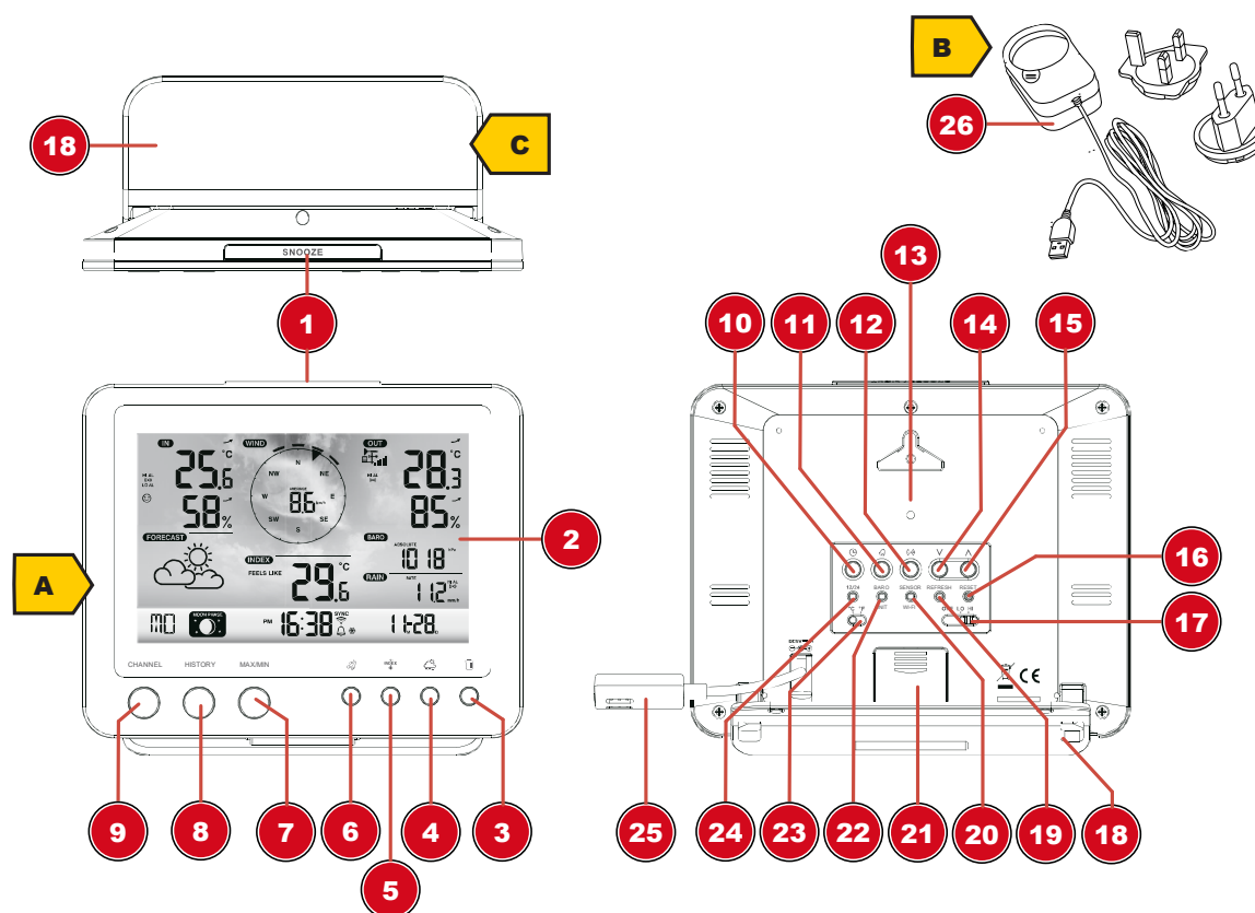
Afb. 1: Alle onderdelen van het basisstation
