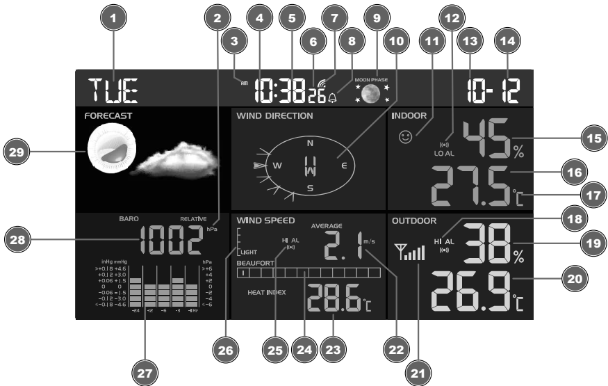
Abb. 2: Display-Anzeigen für die Basisstation
