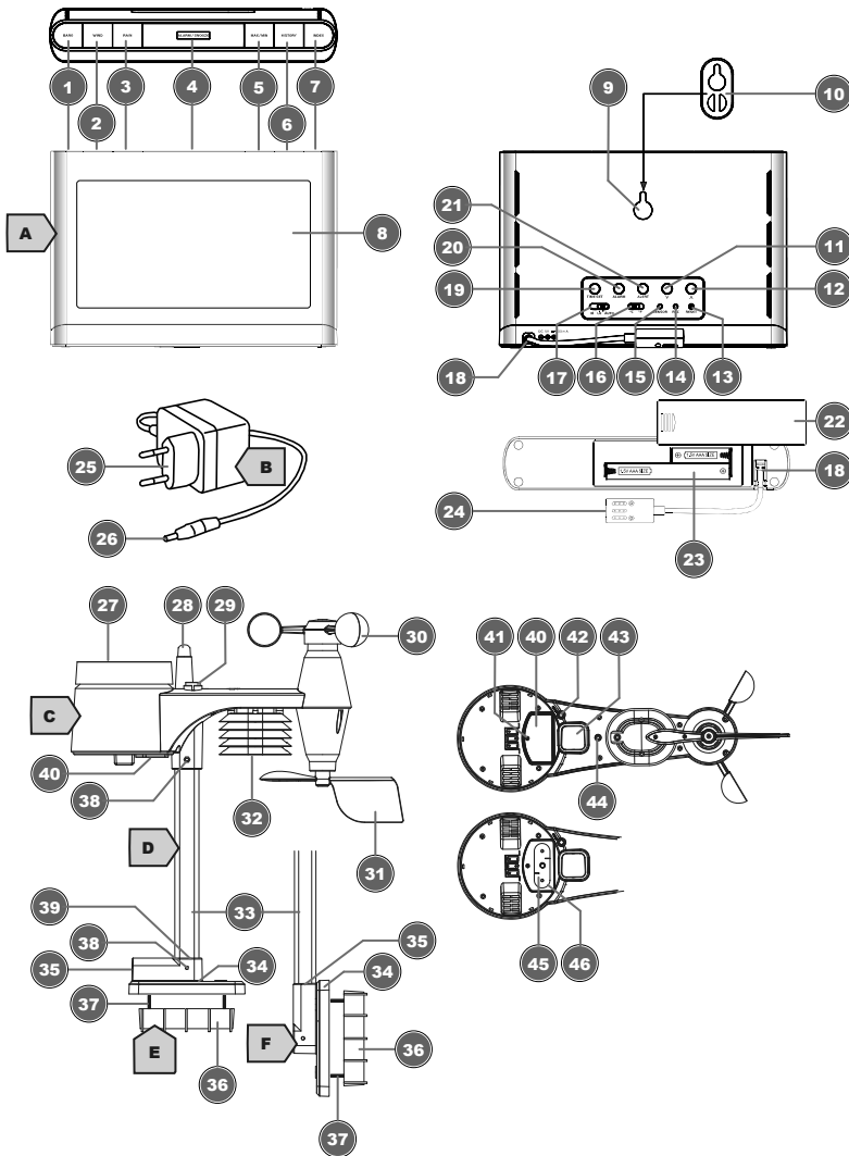
Abb. 1: Teileübersicht für Basisstation (oben) und Funksensor (unten)
